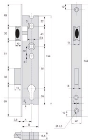
Tête largeur 22
