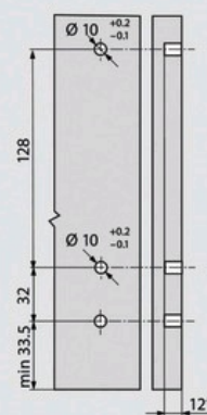
Cotes de perçage de la face pour montage INSERTA/EXPANDO/EXPANDO T et à frapper
