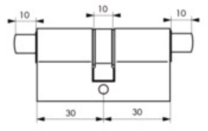
Cylindre profilé avec 2 triangles externes
