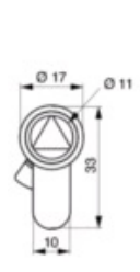
Cylindre profilé avec 2 triangles internes
