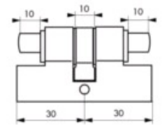
Cylindre profilé avec 2 triangles internes
