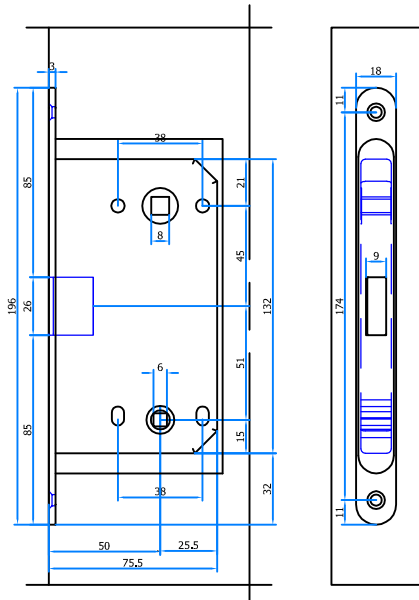
AGB slot WC/badkamer
