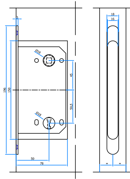
AGB slot cilinder
