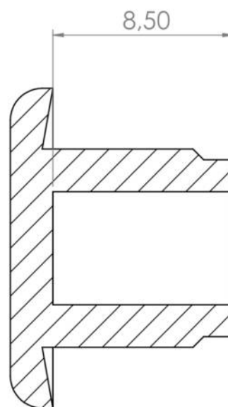
COUPE A-A ECHELLE 4 : 1
