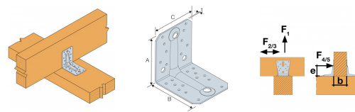
Fixation bois/bois
