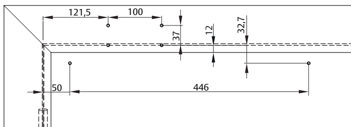
Schéma de fixation pour pose sur l'huissérie côté opposé aux paumelles
