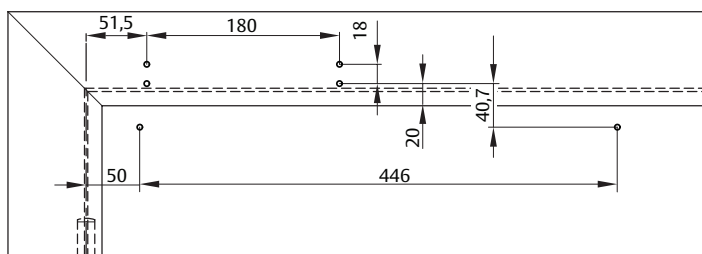
Schéma de fixation sur l'huissérie côté opposé aux paumelles avec plaque de montage
