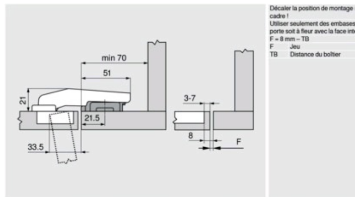
Jeu minimal du jeu F pour faces avec rayon de face (R = 1 mm) selon le réglage d'usine
