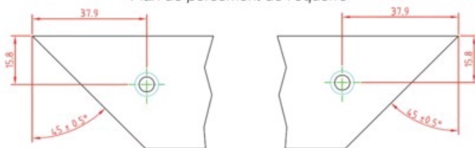
Plan de perçement de l'équerre
