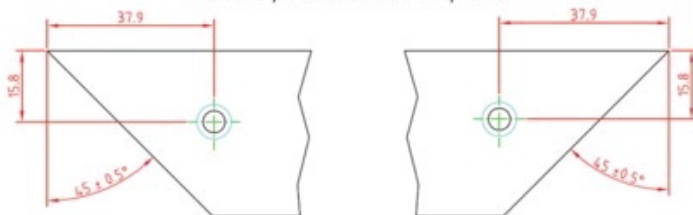
Plan de percement de l'équerre
